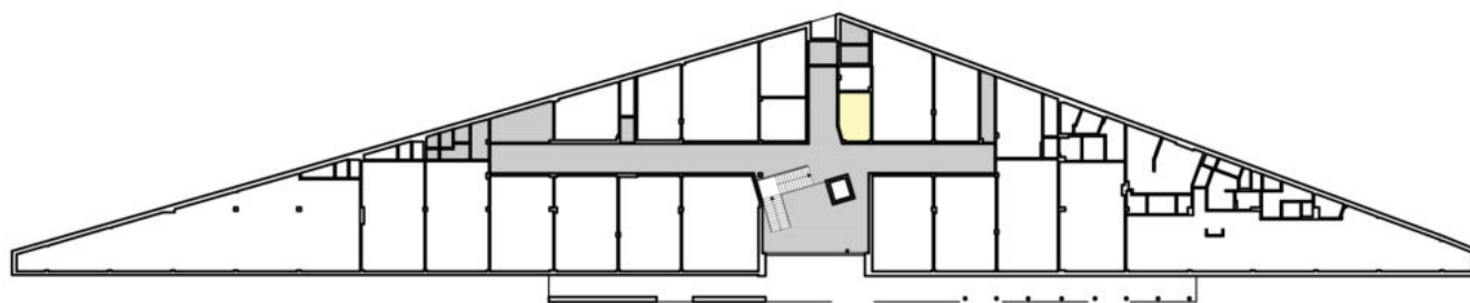
RZUT PARTERU
